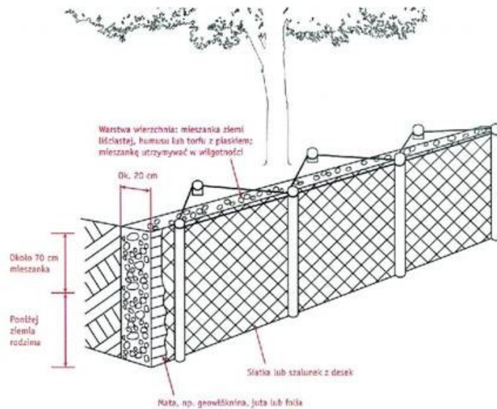
Rys. 1. Budowa zasłony korzeniowej (na podstawie: Szczepanowska 2008).
